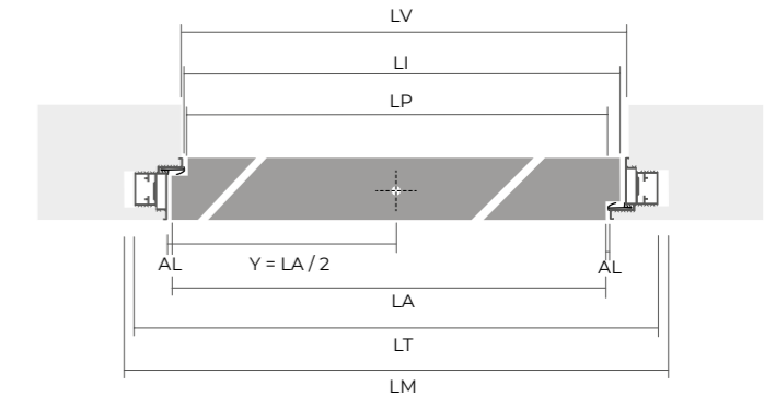
PIVOT CENTRALE central axis
