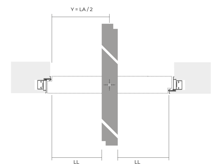
POSIZIONAMENTO PIVOT pivot positioning
